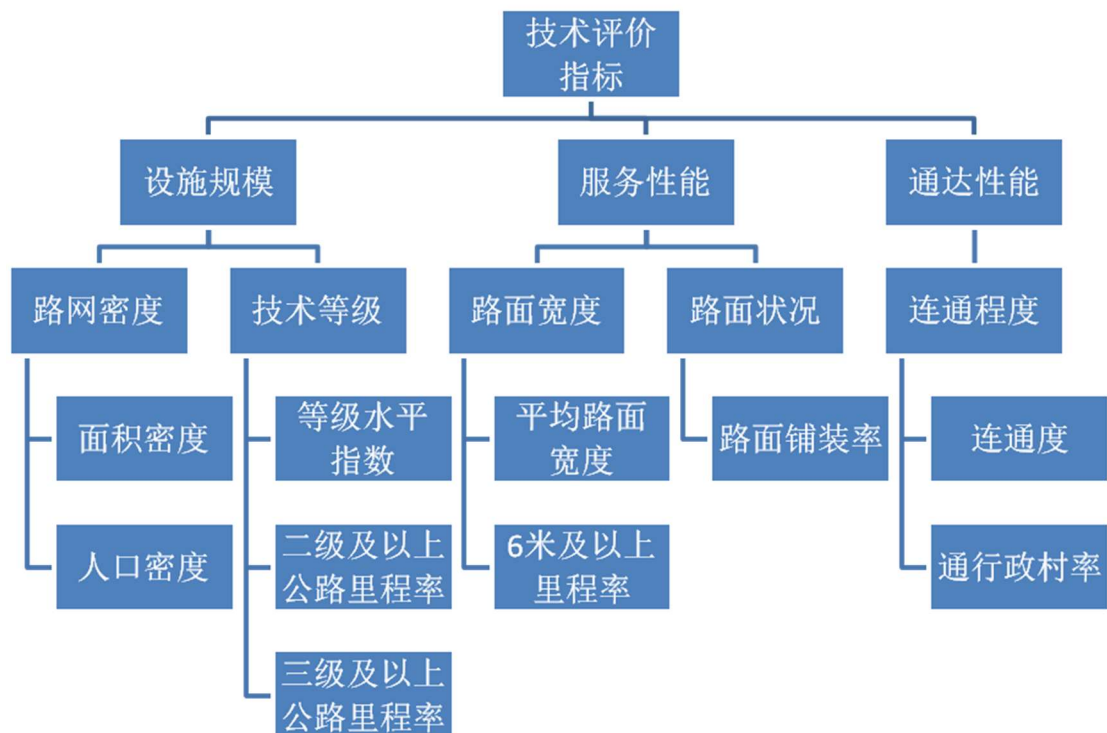
图 2-9 东丽区农村公路技术评价指标体系
